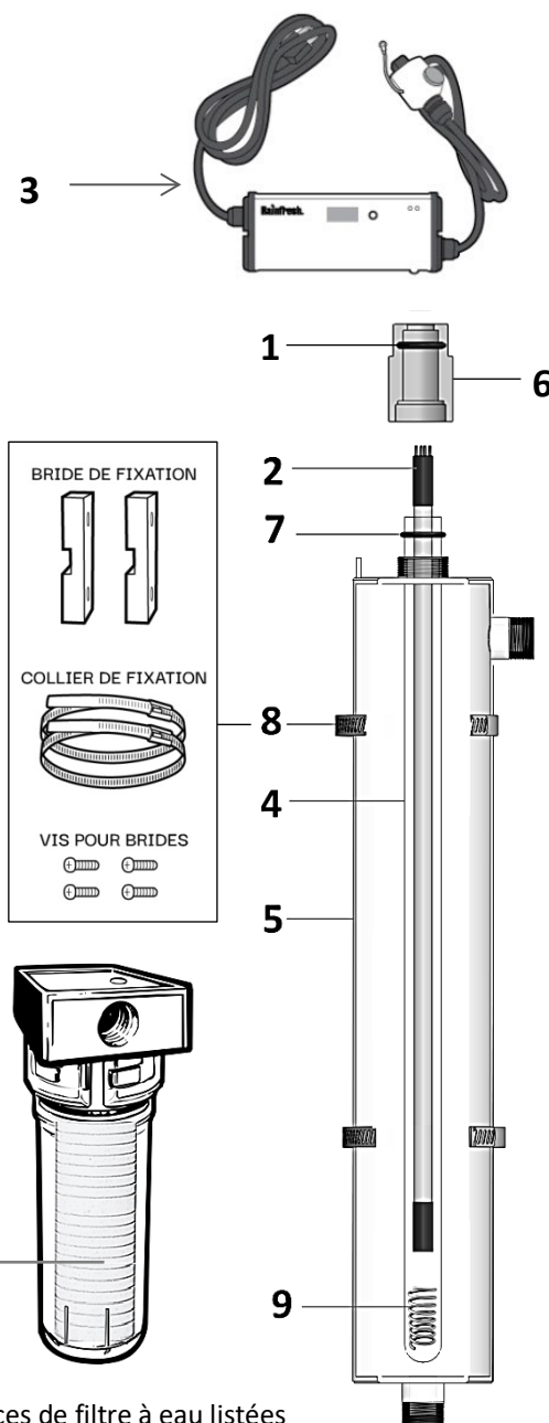
Pièces de filtre à eau listées dans le manuel du filtre (Modèle R830F uniquement)
